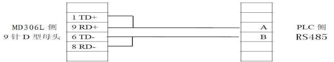
图 3—13 文本通讯线
