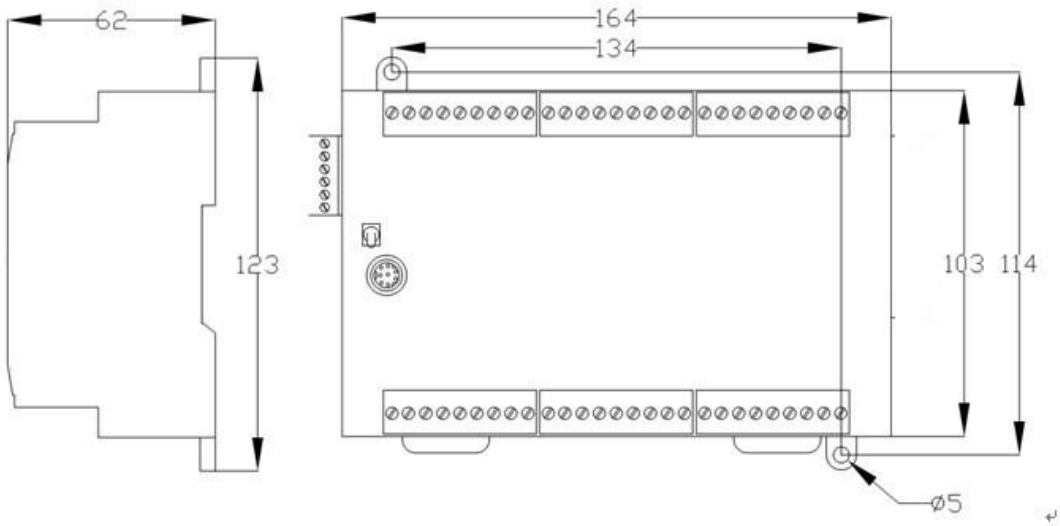
图 2—1.2 TX2N-30 安装尺寸示意图（单位：mm）
