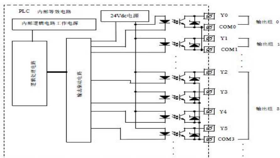
图 3—6 晶体管输出等效电路
