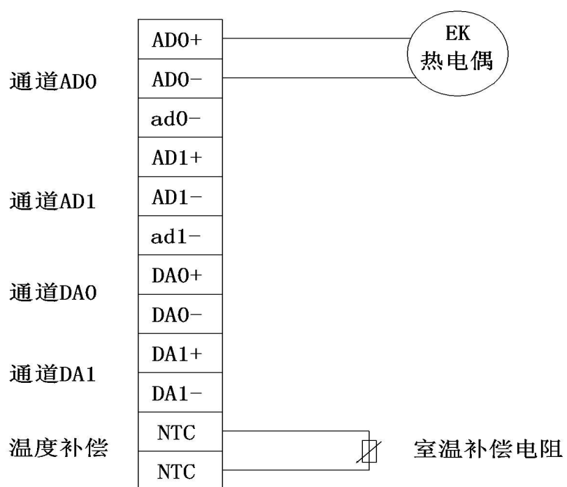
图 3—1 E 型或 K 型热电偶模拟量输入接线方法
