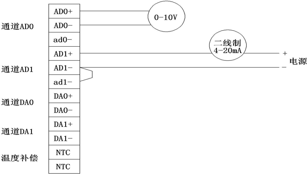
图 3—9 0—10V 和二线制 4-20mA 模拟量输入接线方法
