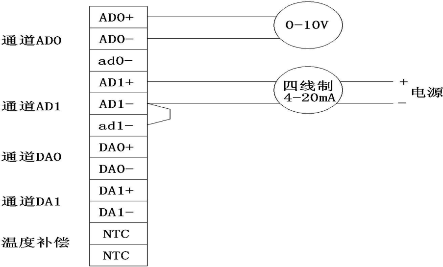
图 3—8 0—10V 和四线制 4-20mA 模拟量输入接线方法
