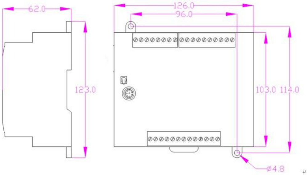
图 2—1.1 TX2N-20 安装尺寸示意图（单位：mm）
