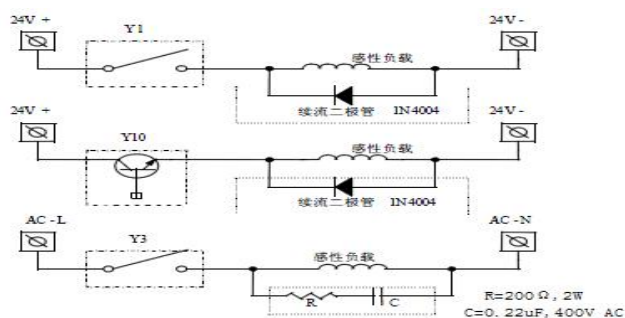
图 3—7 负载保护电路
