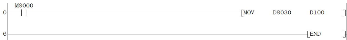
图 3—11 模拟量输入编程示例
