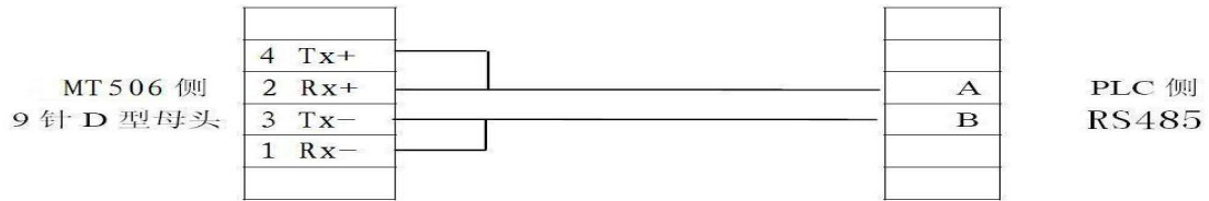
图 3—14 触摸屏通讯线
